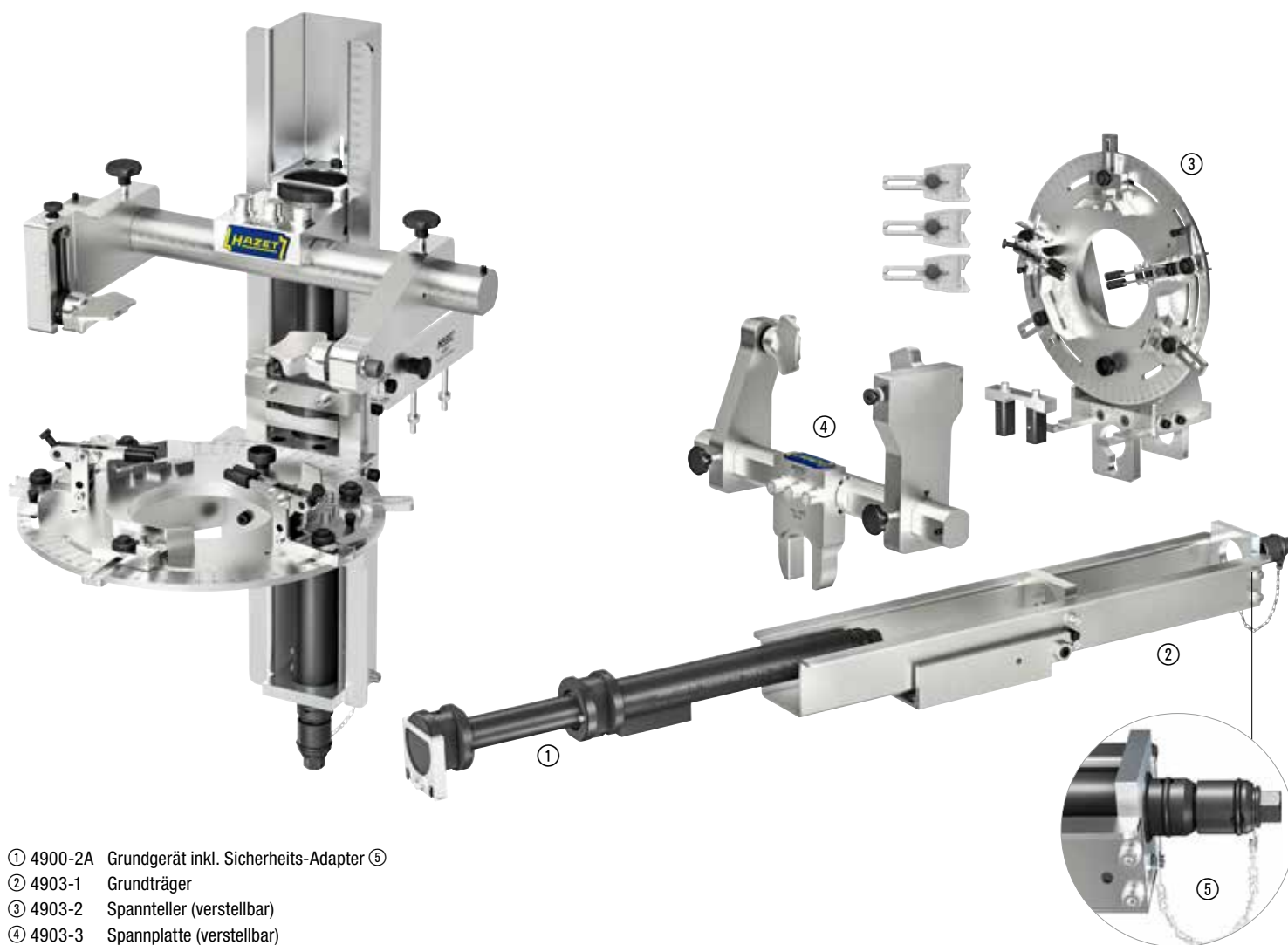
Federbein-Fixierung
