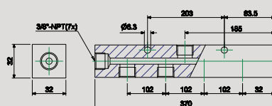
VB401 Verteiler Art.Nr. 7200067
