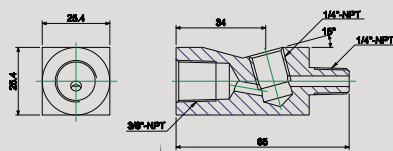
ADG323 T-Stück für Manometer High Flow Art.Nr. 7299232
