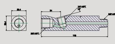
ADT202 T-Stück Art.Nr. 7200202
