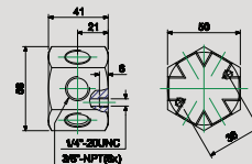
VB66 Regelventil Art.Nr. 7200226
