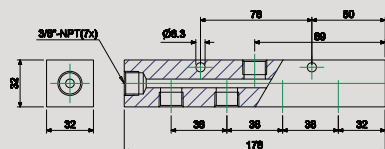
VB201 Verteiler Art.Nr. 7200066
