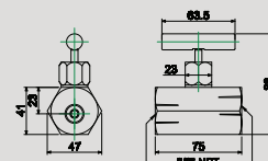
VC331 Regelventil Art.Nr. 7200068
