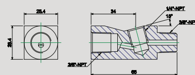
E0567 T-Stück für Manometer Art.Nr. 7299230
