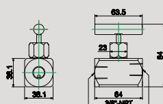
BV42 Sicherheitsventil Art.Nr. 7200342
